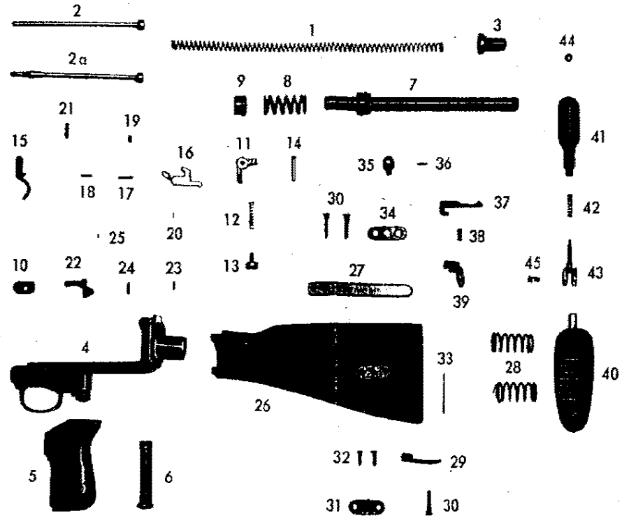
Bodenstück mit Kolben
