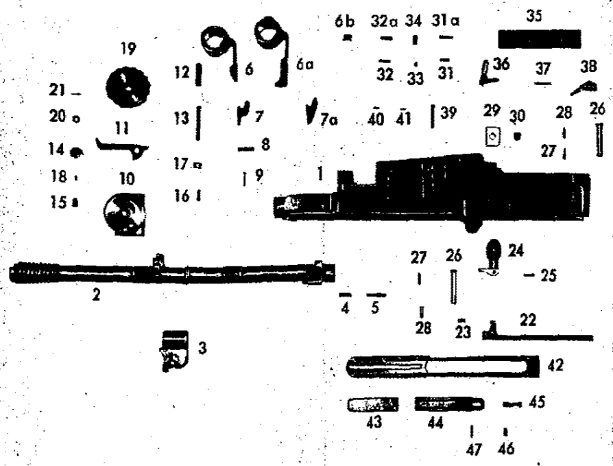
Gehäuse
